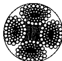
4V × 48S + 5FC 直径 20 ~ 40mm
