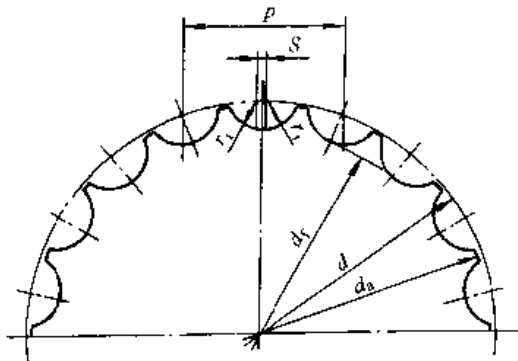
图 8-2-3 齿槽形状
