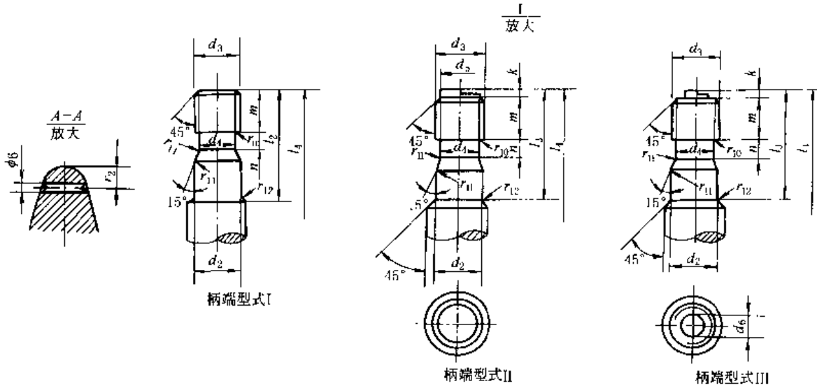
图 8-1-11 直柄单钩
