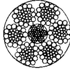
6V × 30 + FWR 直径 20 ~ 38mm
