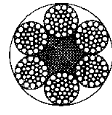
6 × 36SW + FC 直径 12 ~ 60mm
