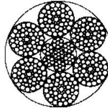
6 × 55SWS + IWR 直径 36 ~ 64mm
