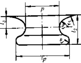
B型铸造圆柱形吊耳
