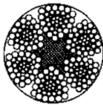
6V × 37S + FC 直径 32 ~ 52mm
