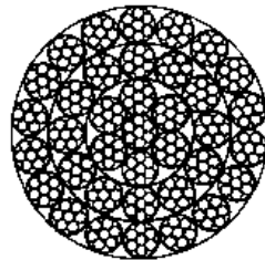
36 × 7 + IWS 直径 16 ~ 44mm
