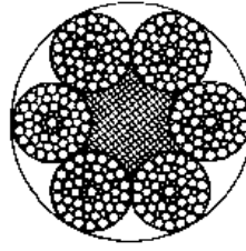
6 × 55SWS + FC 直径 36 ~ 64mm
