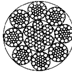
8 × 31SW + IWR 直径 14 ~ 56mm
