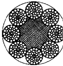
8 × 49SWS + FC 直径 44 ~ 64mm
