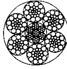
6 × 26SW + IWR 直径 13 ~ 40mm
