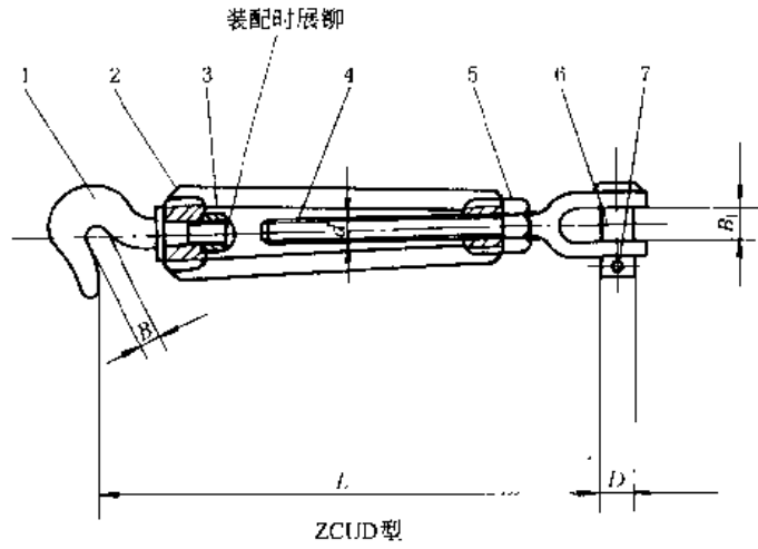
1—钩子；2—模锻螺旋套；3—圆螺母；4—U形螺杆；5—锁紧螺母；6—开口销；7—光直销
