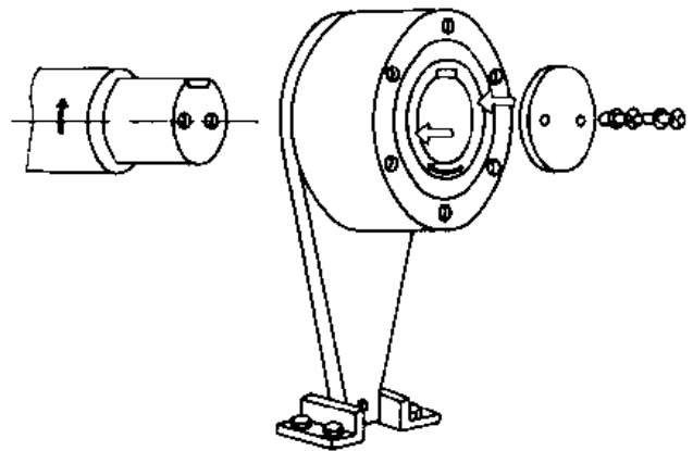
图 8-2-7 安装示意图
