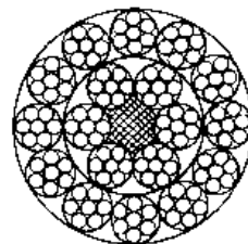
18 × 7 + FC 直径 6 ~ 44mm
