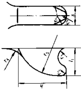
A型铸造钩形吊耳
