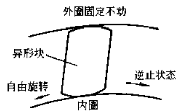
图 8-2-6 原理示意图
