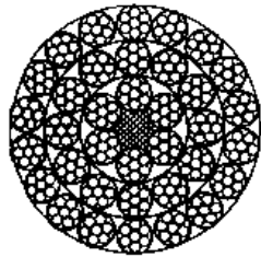
36 × 7 + FC 直径 16 ~ 44mm
