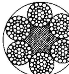
6 × 36SW + IWR 直径 12 ~ 60mm
