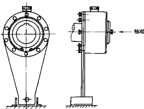
图 8-2-8 NJ(NYD)65 ~ NJ(NYD)200 型逆止器力矩臂圆周限位示意图
