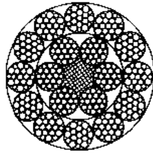
18 × 19W + FC 直径 14 ~ 44mm
