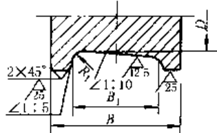
圆锥型踏面尺寸、重量及轨道型号
