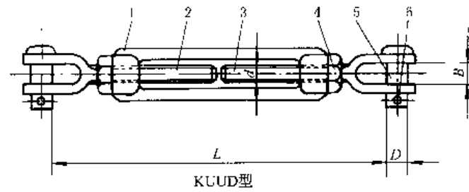
KUUD 型、KUUH 型、KODD 型和 KOOH 型
