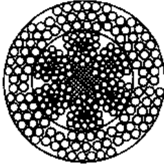
6Q × 19 + 6V × 21 + 7FC 直径 40 ~ 52mm
