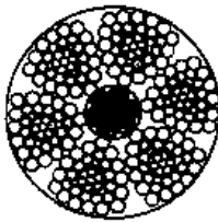
6V × 37S + IWR 直径 32 ~ 52mm
