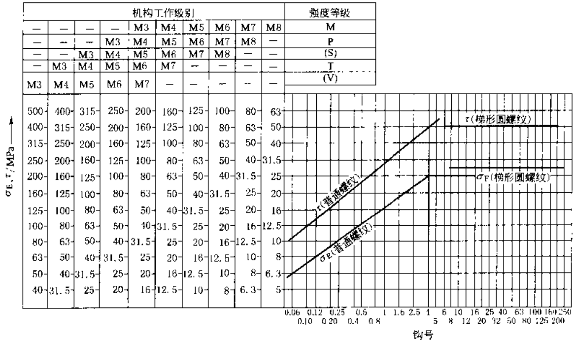
图 8-1-10 单、双钩柄部应力值 \sigma_E 和 \tau (只用于 GB/T 10051.5 规定的单钩尺寸和相应标准规定的双钩尺寸)
