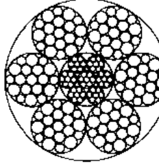
6 × 19W + IWR 直径 11 ~ 40mm
