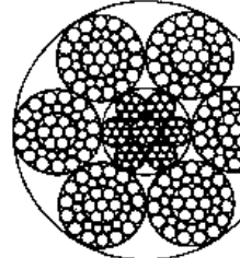
6 × 37S + FC 直径 10 ~ 60mm
