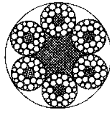
6 × 24W + 7FC 直径 10 ~ 44mm
