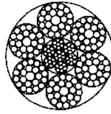
6 × 29Fi + IWR 直径 10 ~ 44mm
