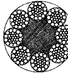
8 × 26SW + IWR 直径 16 ~ 48mm
