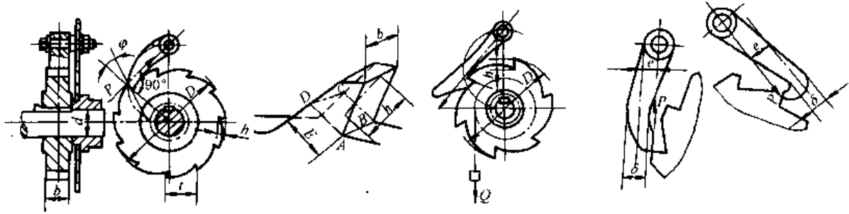
图 8-1-12 棘轮
