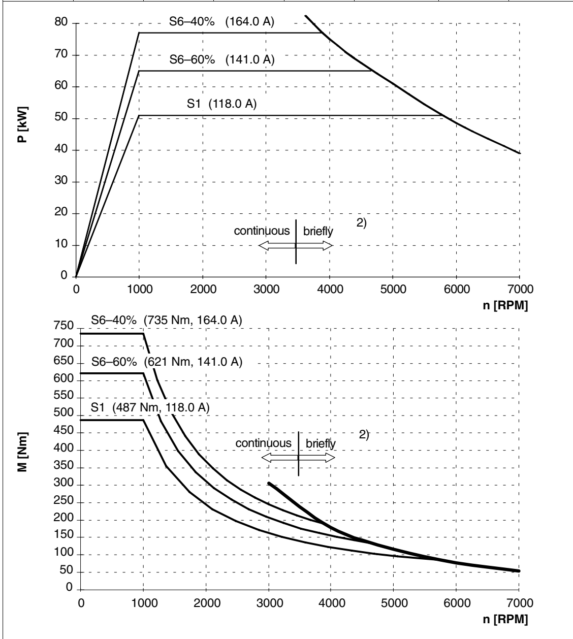
Fig. 2-55 1PH7186-□ND□□
