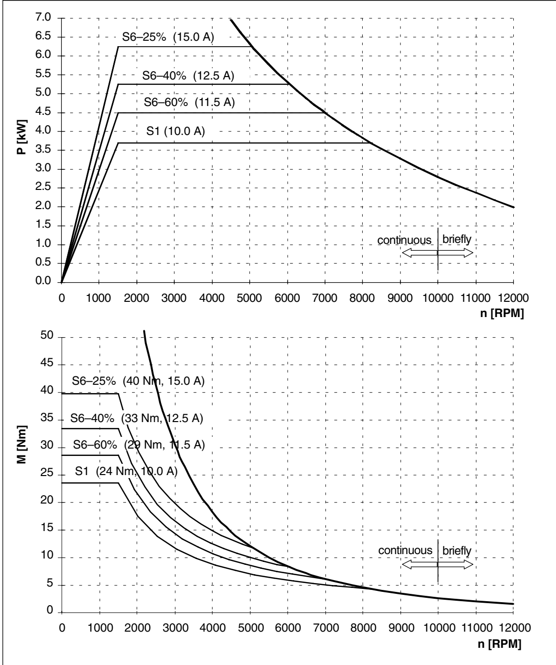
Fig. 2-2 1PH7101-□NF□□-0L
