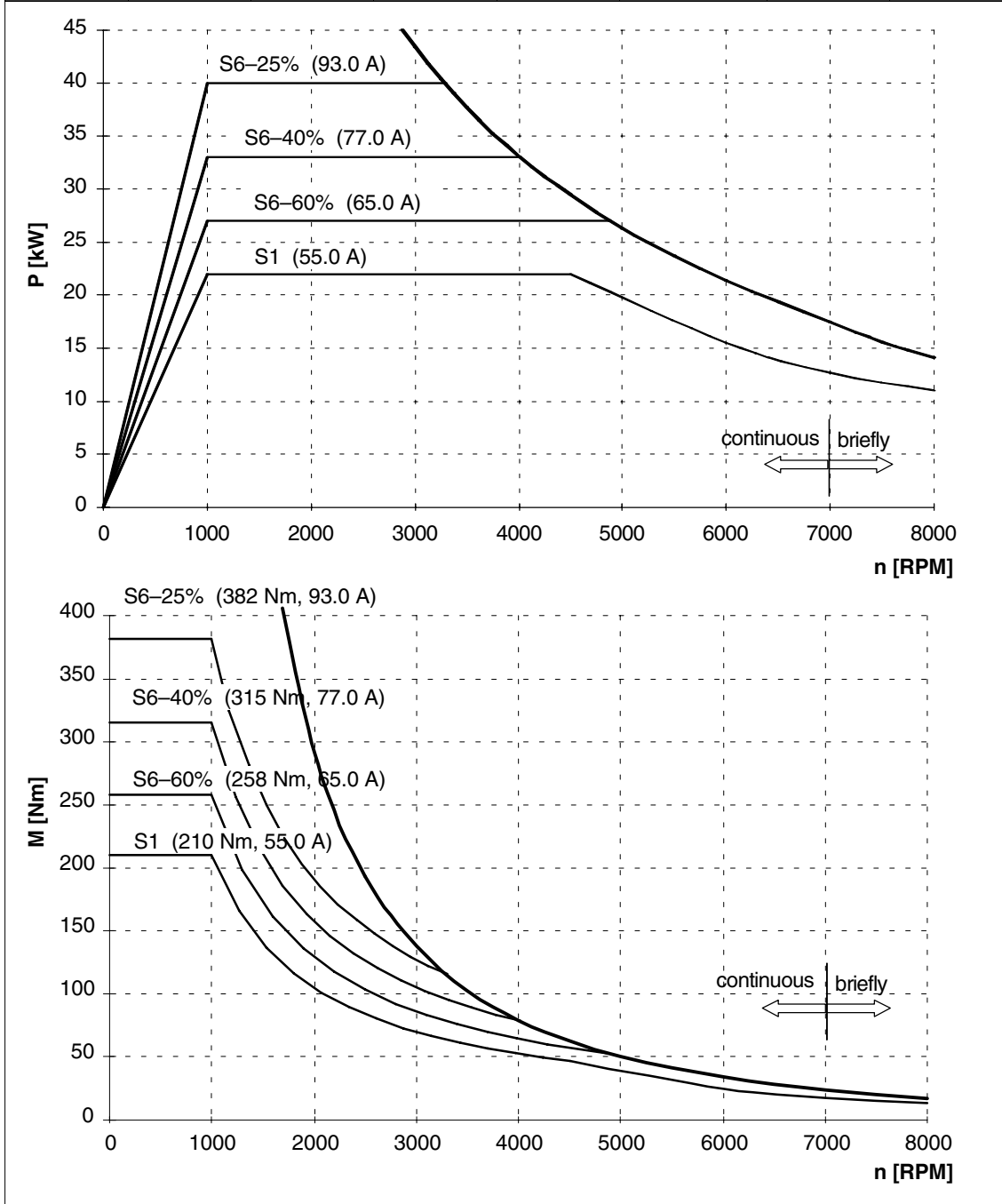
Fig. 2-36 1PH7163-□ND□□-0L
