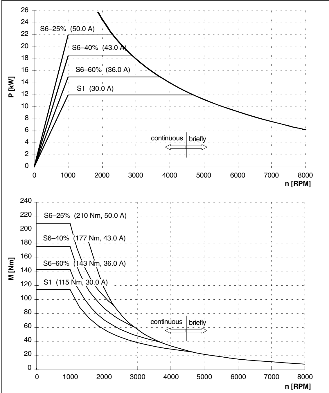
Fig. 2-19 1PH7133-□ND□□
