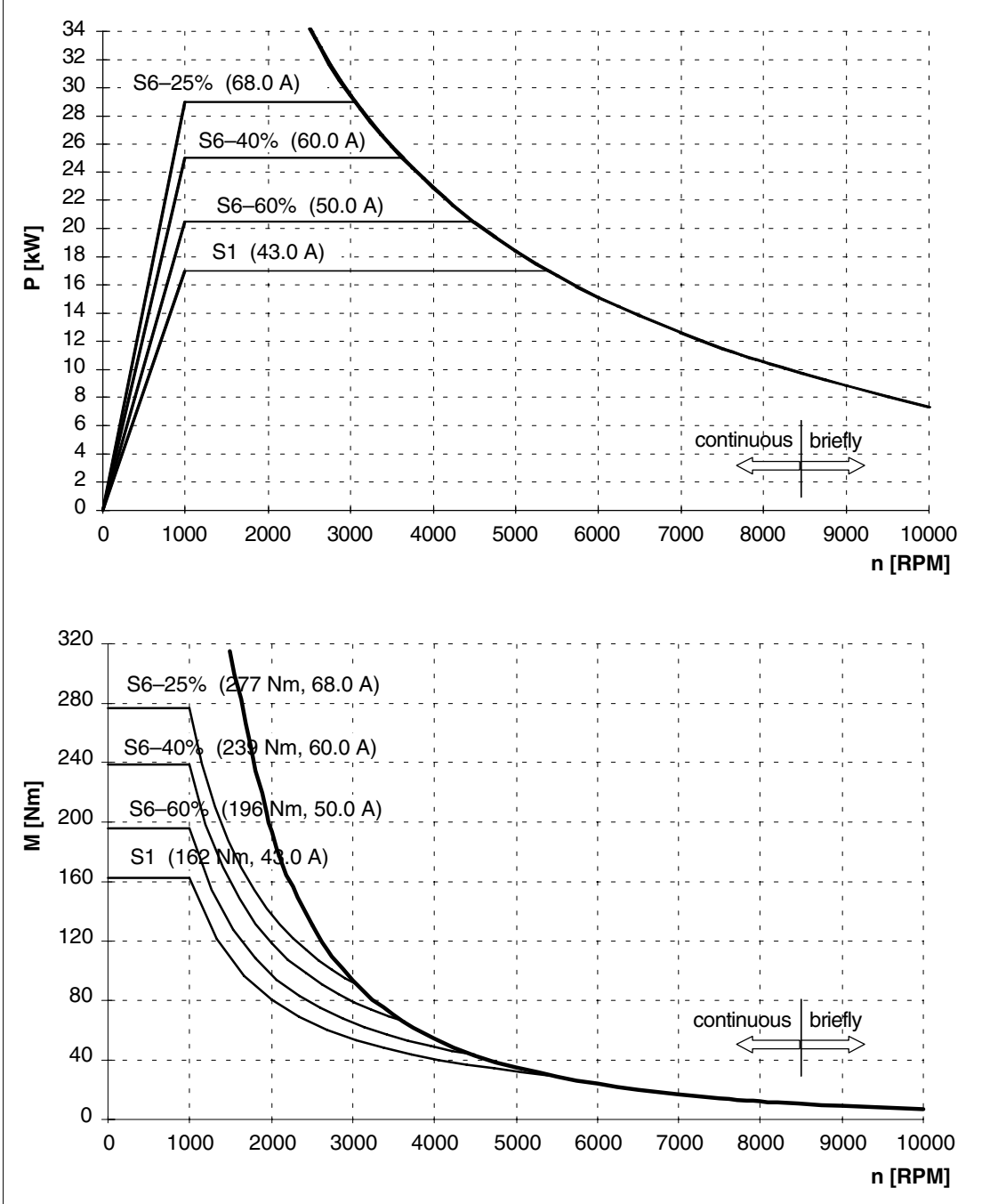
Fig. 2-28 1PH7137-□ND□□-0L
