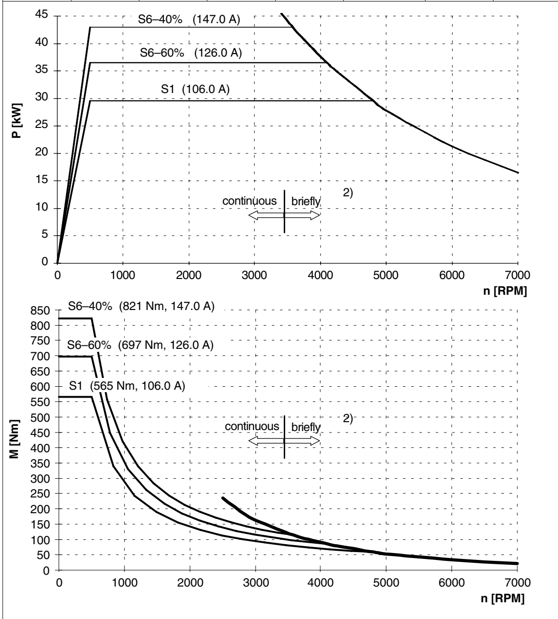
Fig. 2-54 1PH7186-□NT□□
