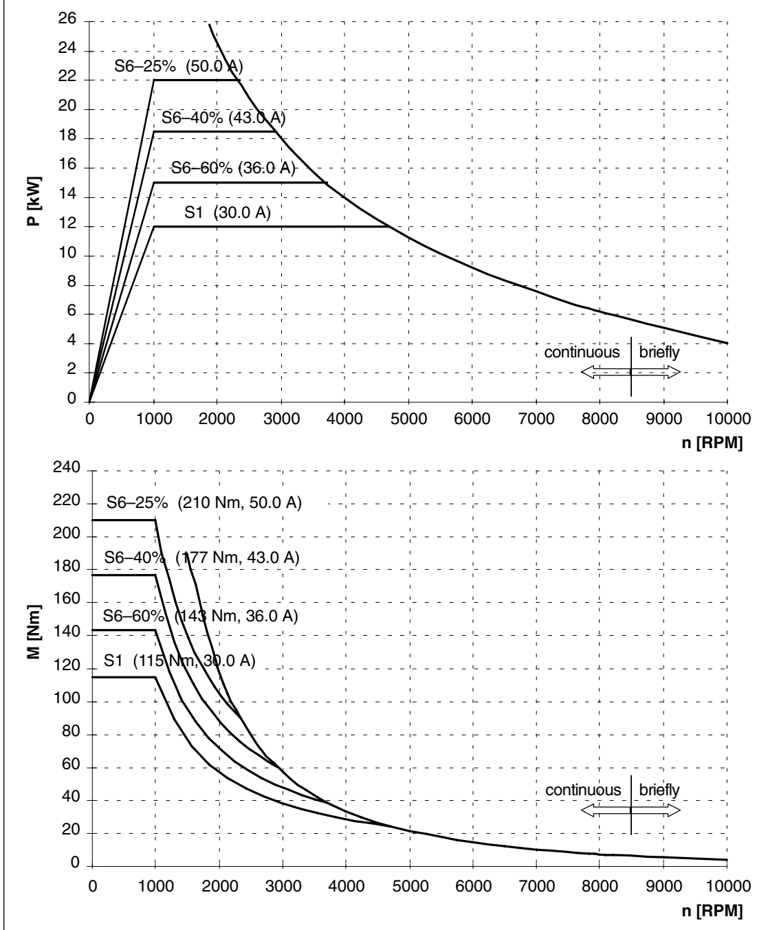
Fig. 2-20 1PH7133-ND-OL
