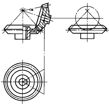
图 17 轴线斜交的锥齿轮副的啮合画法
