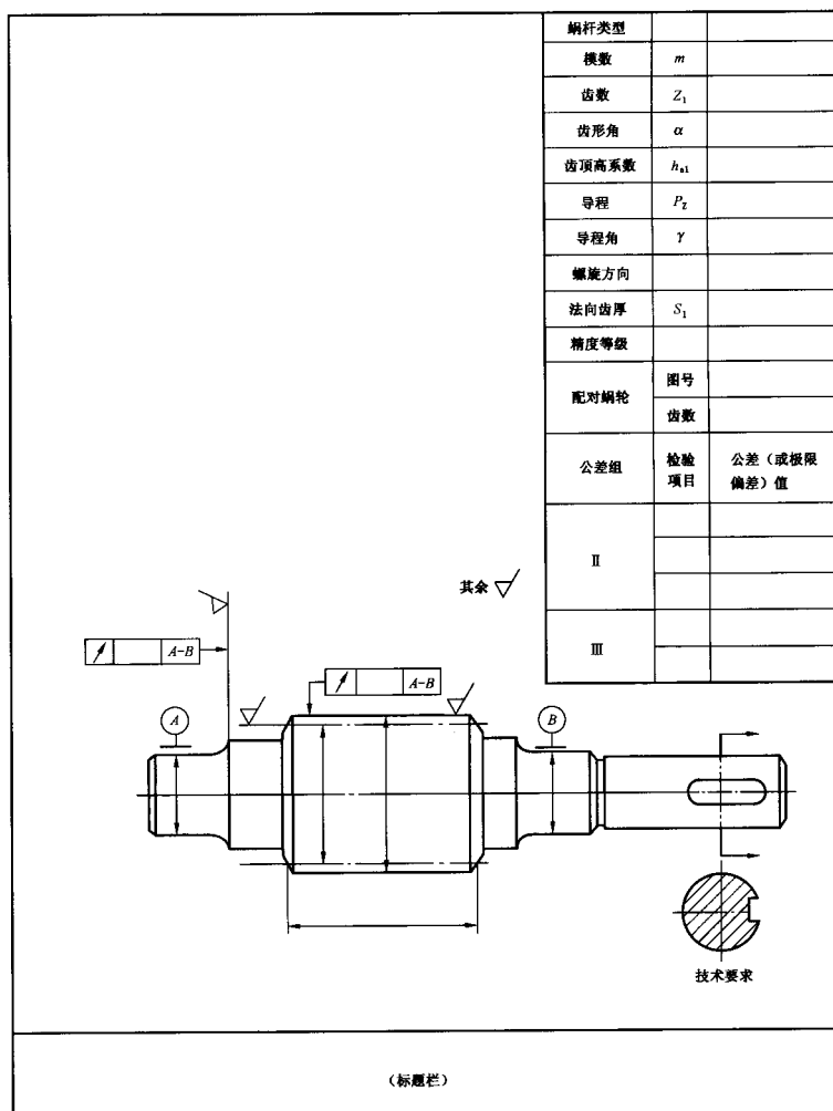
图 A.3 蜗杆图样格式示例
