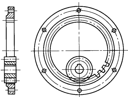
图 11 圆柱齿轮副的啮合画法——内啮合
