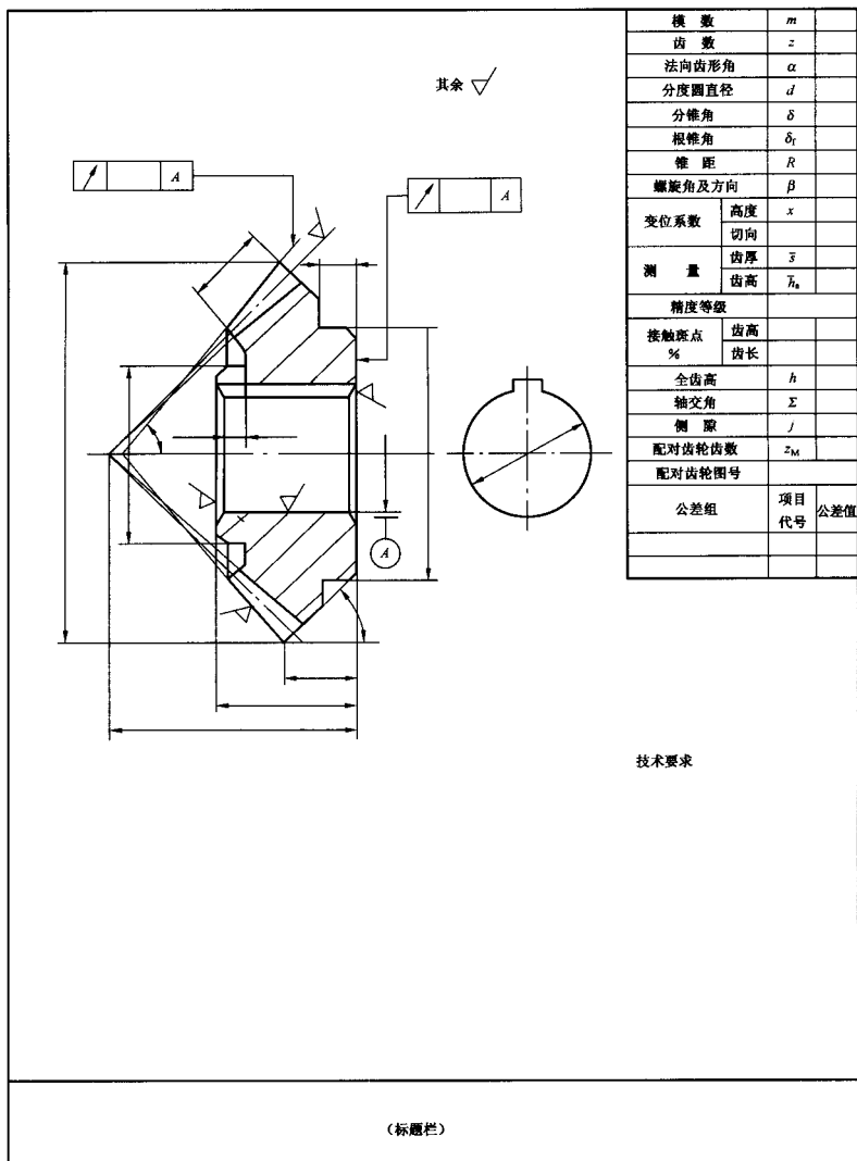
图 A.2 锥齿轮图样格式示例
