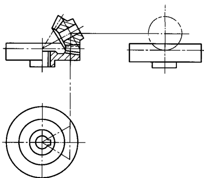
图 18 轴线斜交的平面齿轮与锥齿轮的啮合画法
