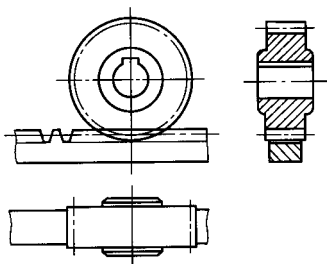
图 12 齿轮齿条副的啮合画法
