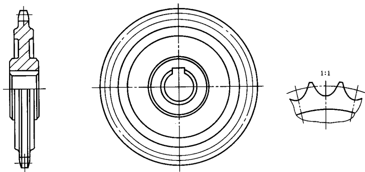
图7 链轮画法
