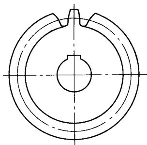
图5 表明齿形的圆柱齿轮画法
