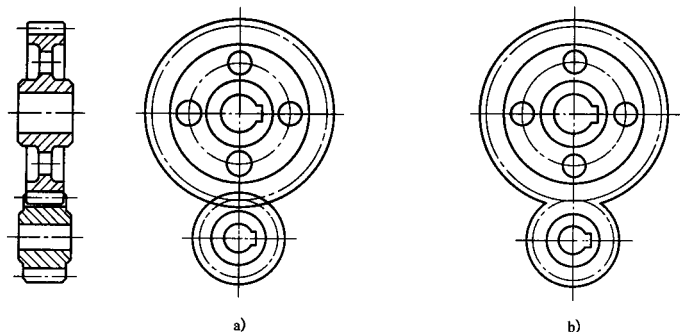
图9 圆柱齿轮副的啮合画法——外啮合(一)
