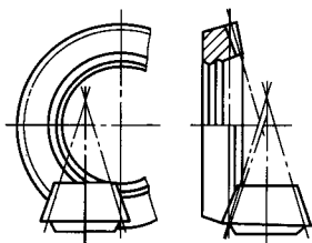
图 15 准双曲面齿轮副的啮合画法
