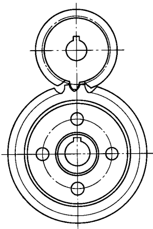
图 24 圆弧齿轮副的啮合画法
