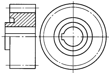
图 1 圆柱齿轮画法
