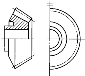
图 2 锥齿轮画法
