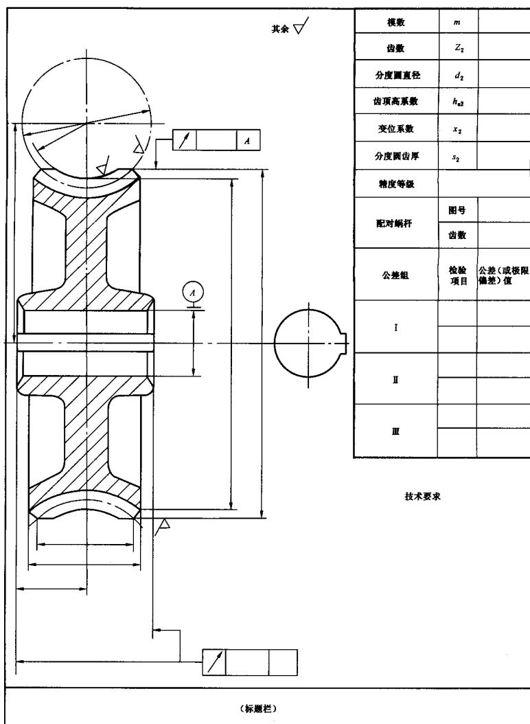
图 A.4 蜗轮图样格式示例
