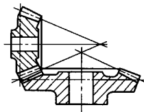
图 16 八字啮合锥齿轮副的啮合画法
