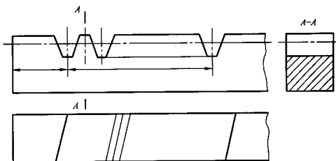
图4 齿条画法
