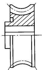
图3 蜗轮画法
