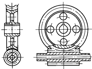
图 22 圆柱蜗杆副的啮合画法(二)
