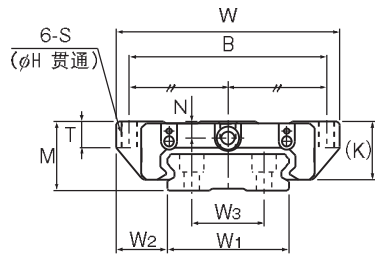
SHW17CAM型、SHW21~50CA型
