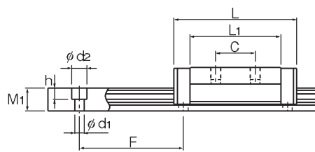
SHW17CRM型、SHW21CR型
