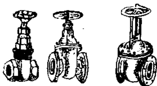
内螺纹连接 法兰连接 法兰连接 暗杆楔式单闸板 明杆平行双闸板
